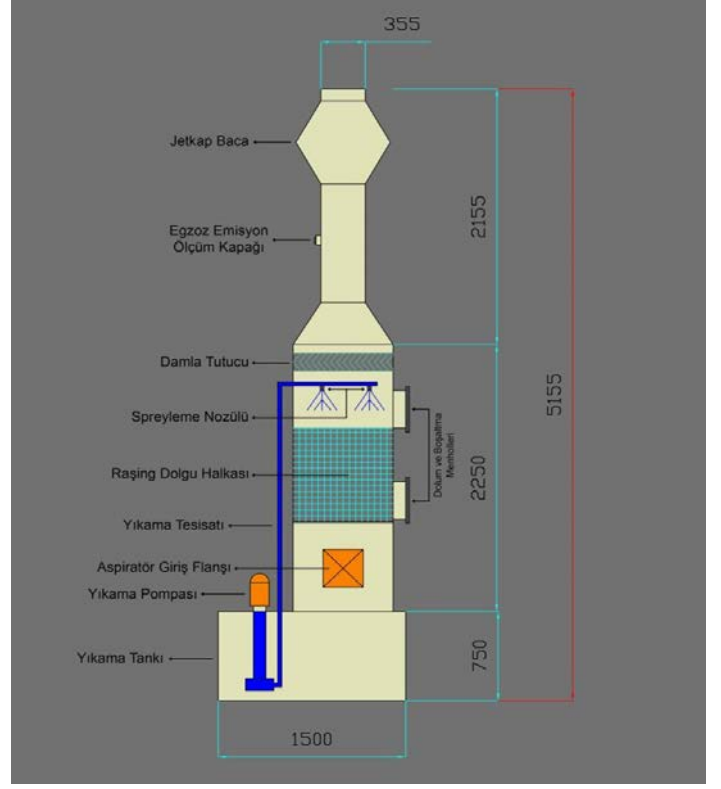
SUCRUBER TEKNİK ÇİZİMİ
